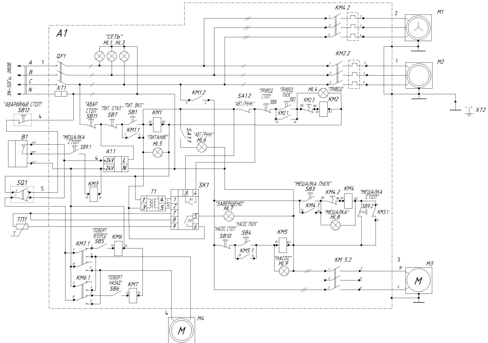
Рисунок 6. Куттер ИПКС-032-80(Н); ИПКС-032-80П(Н) ИПКС 032-80.16.00.000-01 ЭЗ.
