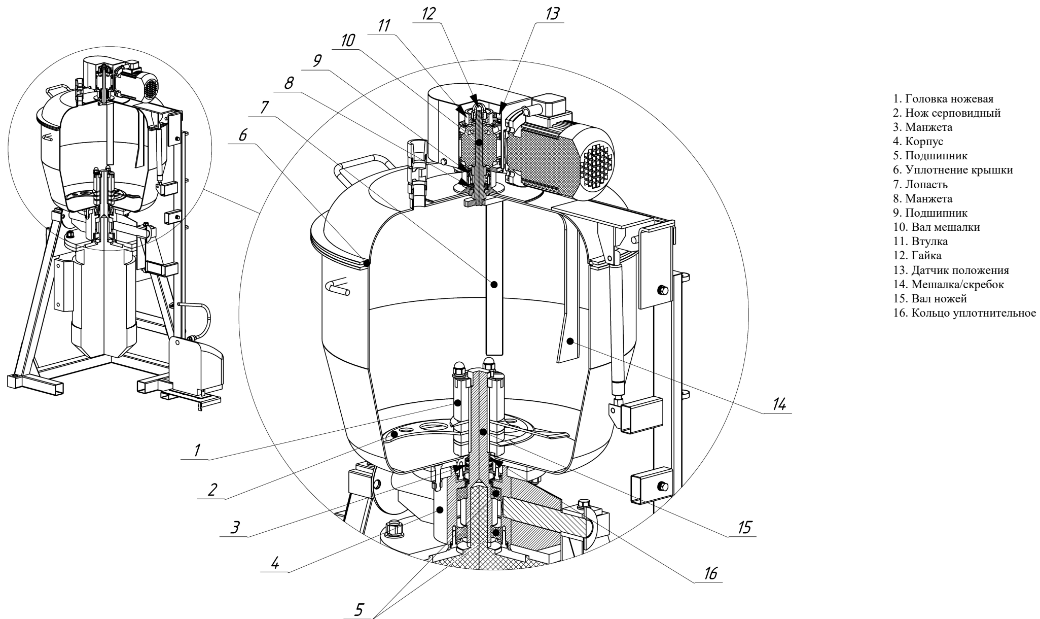
Рисунок 3. Куттер ИПКС-032-80(Н); ИПКС-032-80Р(Н); ИПКС-032-80П(Н); ИПКС-032-80ПП(Н). Внутреннее устройство
